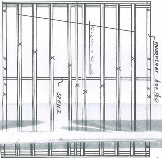
VOOR-GEVEL
